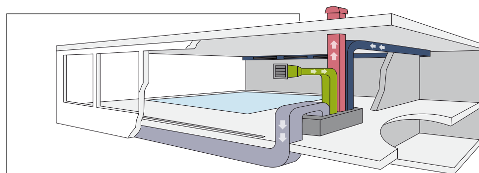
Deumidificazione della piscina interna TOPRAS con sterilizzazione dell'aria integrata
