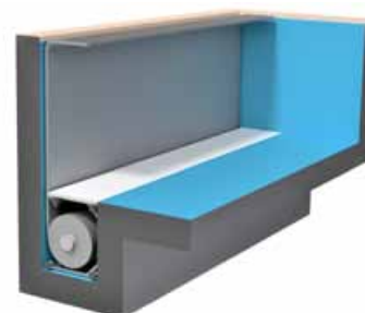
Nascosto in un vano a pavimento
