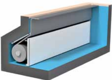
Vano adiacente alla vasca con separazione in pannelli Topras
